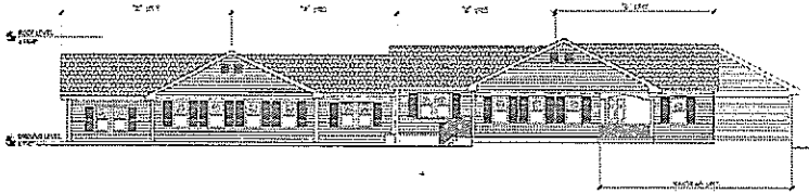
2 REAR ELEVATION SCALE: 1/8" = 1'-0"
